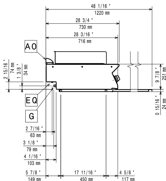
Oldalnézet
